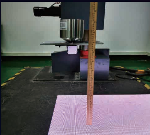
Drop test 1k10
